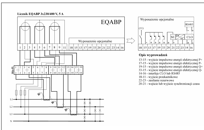
Przykładowy schemat podłączenia
