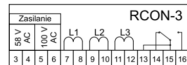
Widok listwy zaciskowej
