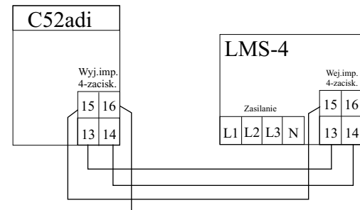
Indukcyjny licznik energii elektrycznej np. C52adi z wyjściem impulsowym 4-zaciskowym
