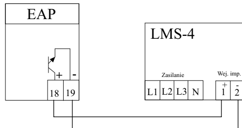
Elektroniczny licznik energii elektrycznej z wyjściem impulsowym typu OC
