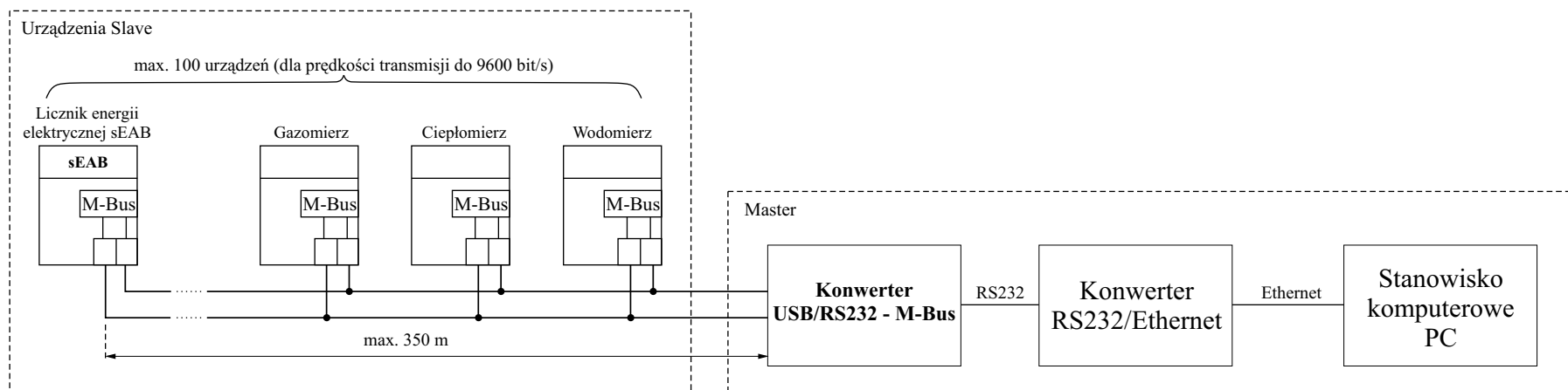
Maksymalne długości przewodu magistrali M-Bus
