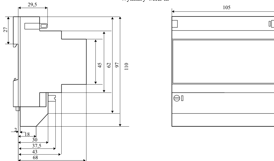
Wymiary MKi-m
